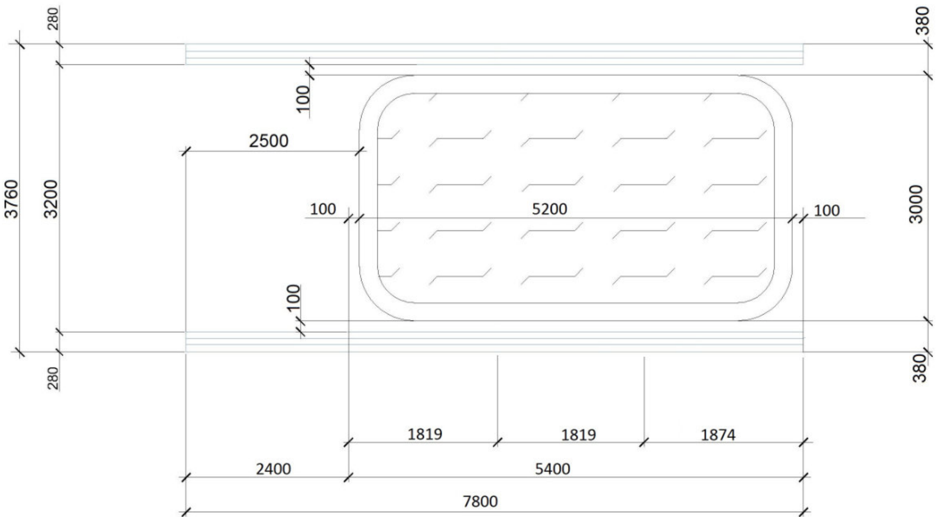
plan sekcji
