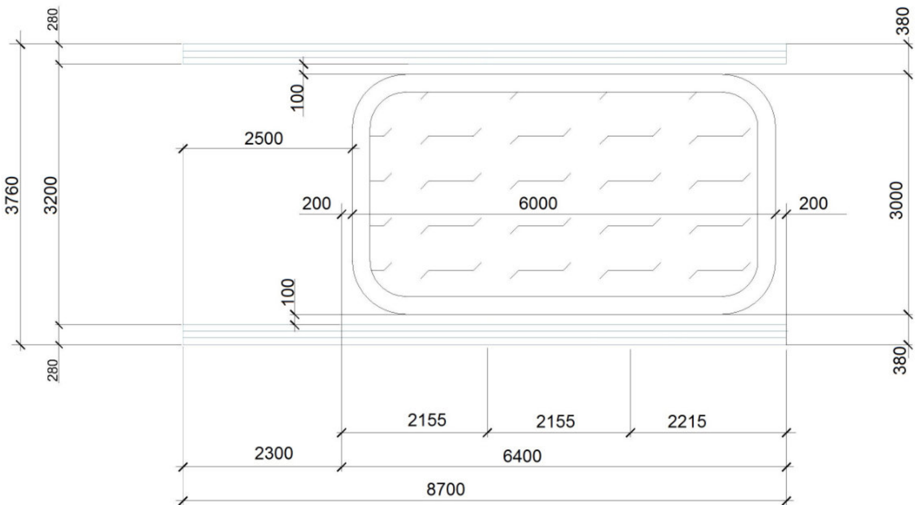
plan sekcji
