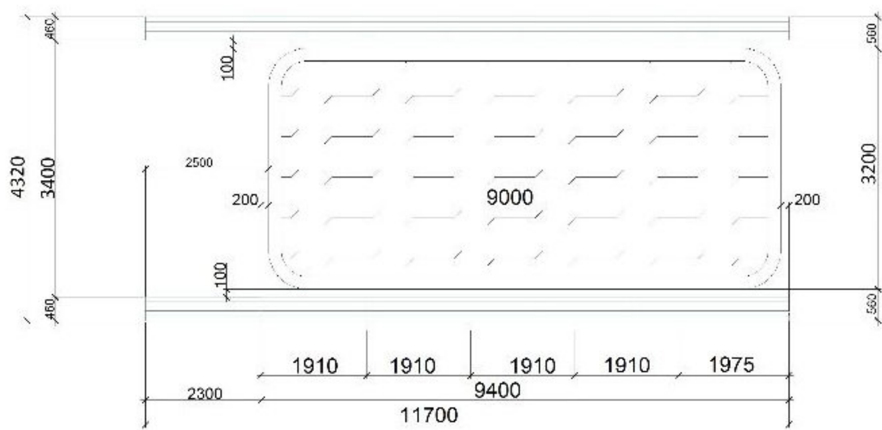
plan sekcji
