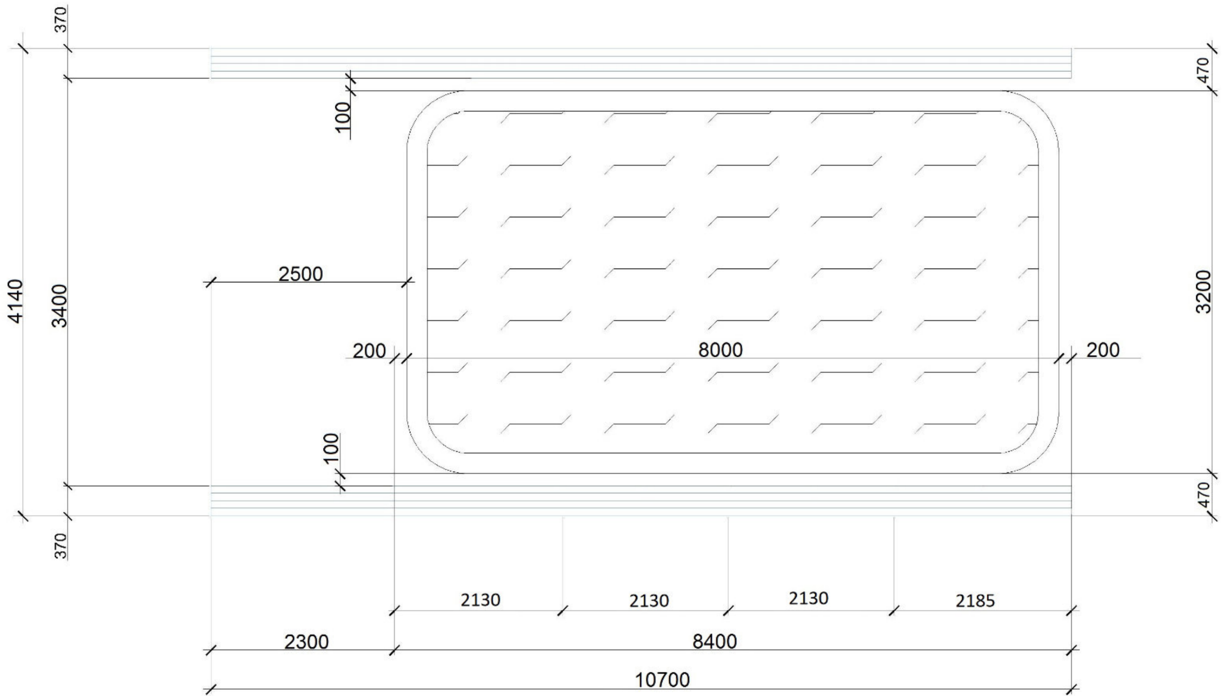
plan sekcji
