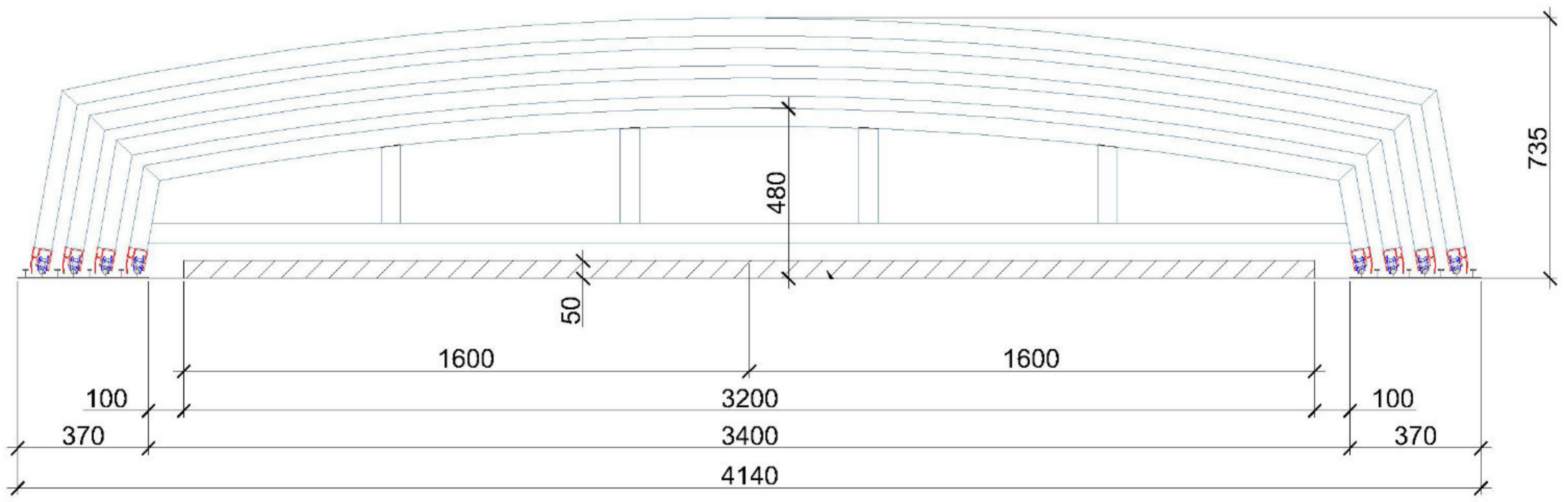
plan sekcji
